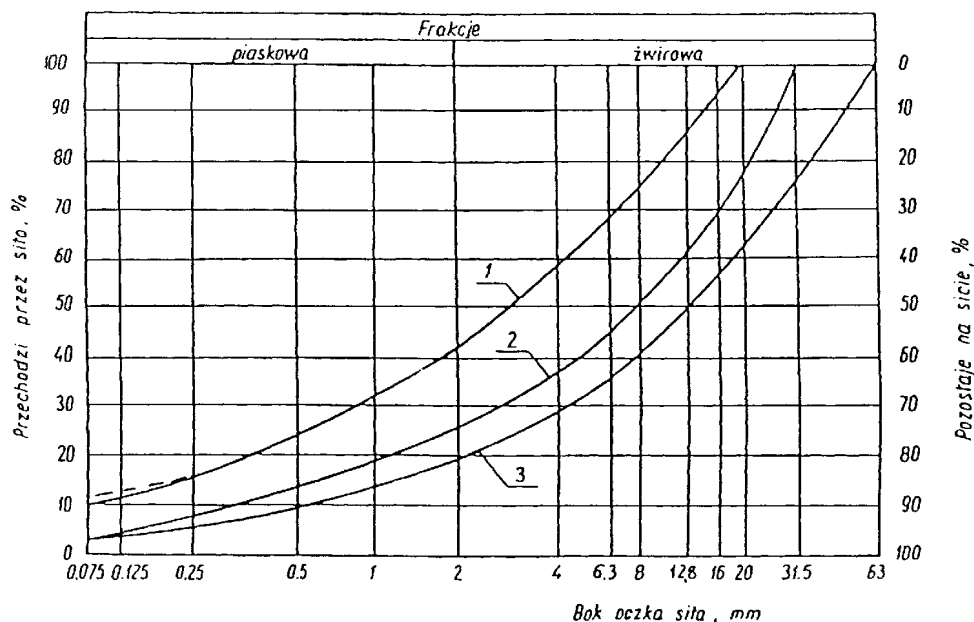
Rysunek 1. Pole dobrego uziarnienia kruszywa przez znaczonych na podbudowy
