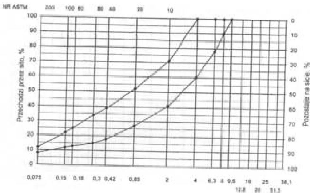
Rys.1 Krzywe graniczne uziarnienia mieszanki mineralnej BA od 0 do 8 mm, od 0 do 6,3 mm do warstwy ścieralnej nawierzchni drogi o obciążeniu ruchem nawierzchni drogi o obciążeniu ruchem KR 1 lub KR 2
